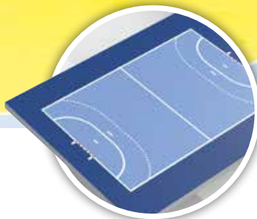
ГАНДБОЛ
